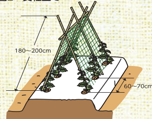
図2 支柱立て
